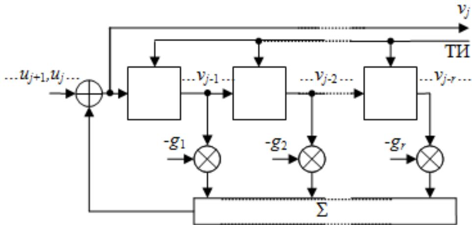
Рис. 2.11 – Рекурсивный цифровой фильтр
