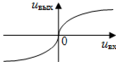
Рис. 2.9 – Амплитудная характеристика компрессора
