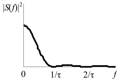
Рис. 2.14 – Спектр плотности мощности последовательности двоичных импульсов
