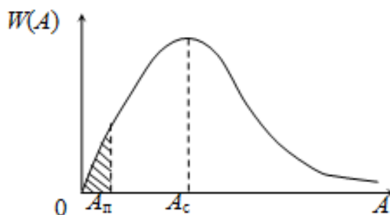
Рис. 5.9 – Релеевское распределение вероятности амплитуды сигнала
