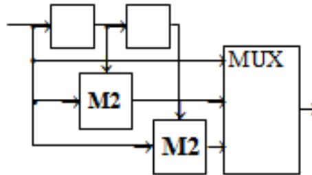
Рис. 3.7 – Схема кодера систематического сверточного кода для k/n = 1/3
