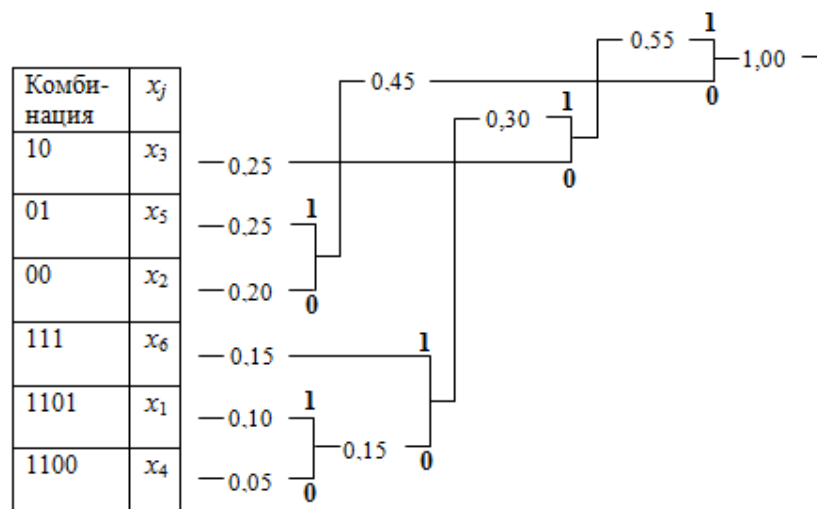
Рис. 4.2 – Кодовое дерево кода Хаффмана
