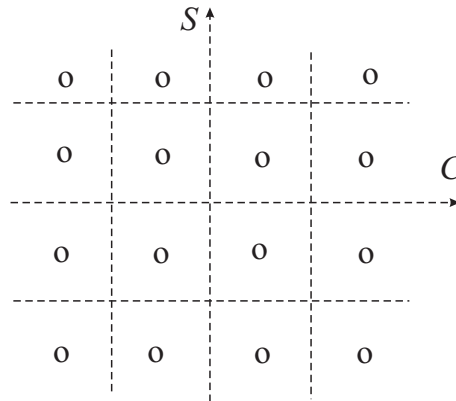
Рис. 5.3 – Подмножества, соответствующие каждому из сигналов КАМ-16
