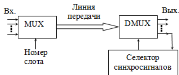
Рис. 6.3 – Принципиальные элементы СПИ с ВРК
