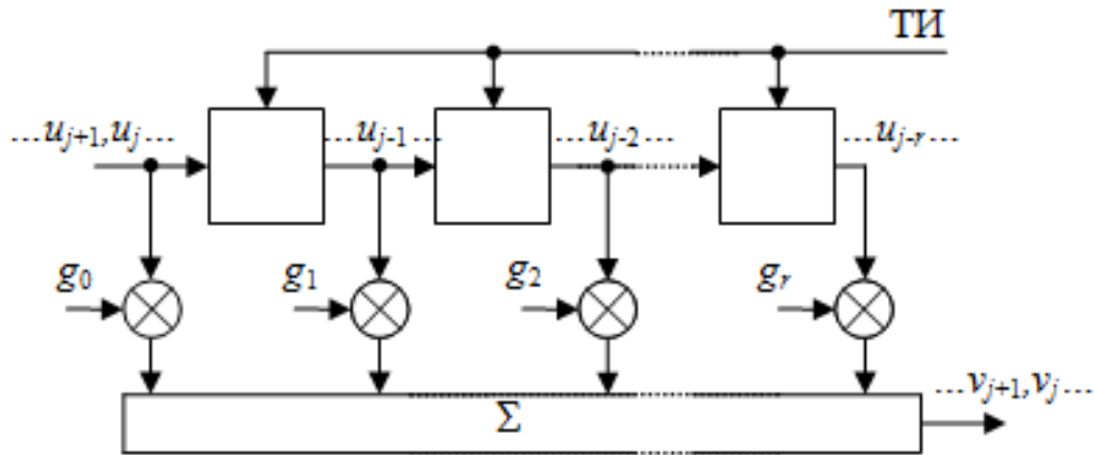
Рис. 2.10 – Трансверсальный цифровой фильтр
