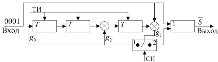
Рис. 3.4 – Кодер циклического кода
