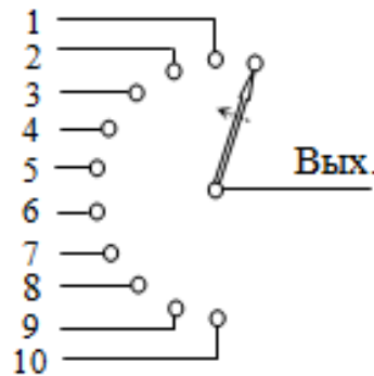
Рис. 7.3 – Схема декадно-шагового искателя
