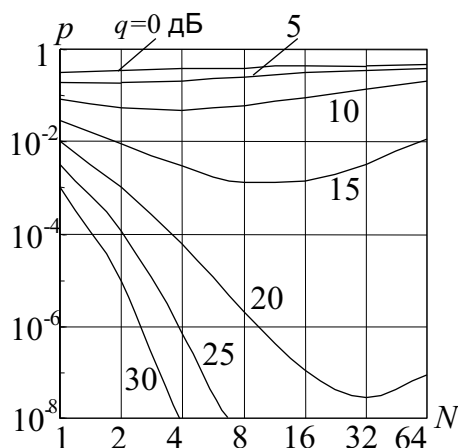
Рис. 5.10 – Зависимость битовой вероятности ошибки при различении двух равновероятных ортогональных сигналов от кратности разнесения при различных значениях отношения сигнал/шум
