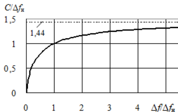
Рис. 4.6 – Пропускная способность непрерывного канала с белым шумом
