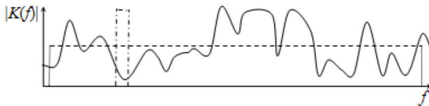
Рис. 6.9 – Примеры «мгновенной» амплитудно-частотной характеристики канала с частотно-селективными замираниями (сплошная линия), спектров узкополосного (штрих-пунктир) и широкополосного (штрих) сигналов
