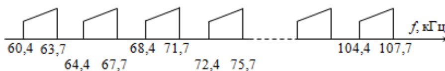
Рис. 6.5 – Спектр первичного группового сигнала
