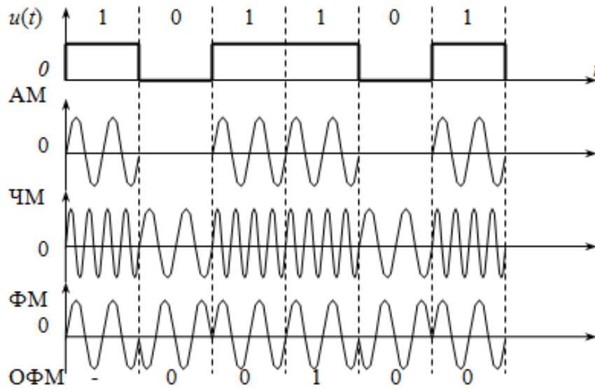
Рис. 2.13 – Методы модуляции гармонической несущей последовательностью двоичных символов
