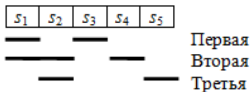
Рис. 3.1 – Схема проверок на чётность для кода (5, 2)
