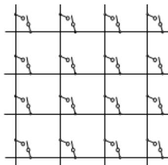
Рис. 7.4 – Схема многократного координатного соединителя
