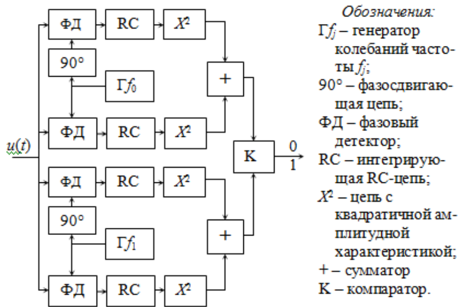
Рис. 5.4 – Функциональная схема демодулятора некогерентного сигнала с ЧМ
