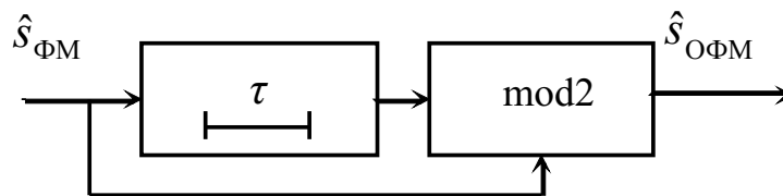
Рис. 5.7 – Схема сравнения решений, вынесенных по соседним импульсам
