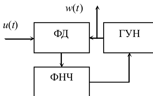
Рис. 5.5 – Генератор опорного колебания с петлей ФАПЧ
