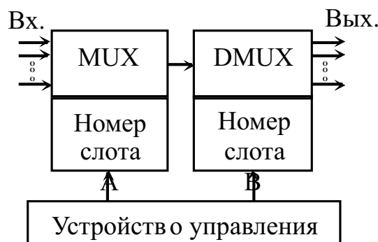
Рис. 7.5 – Схема коммутатора временных интервалов
