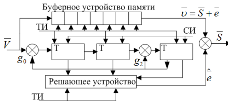
Рис. 3.5 – Декодер циклического кода
