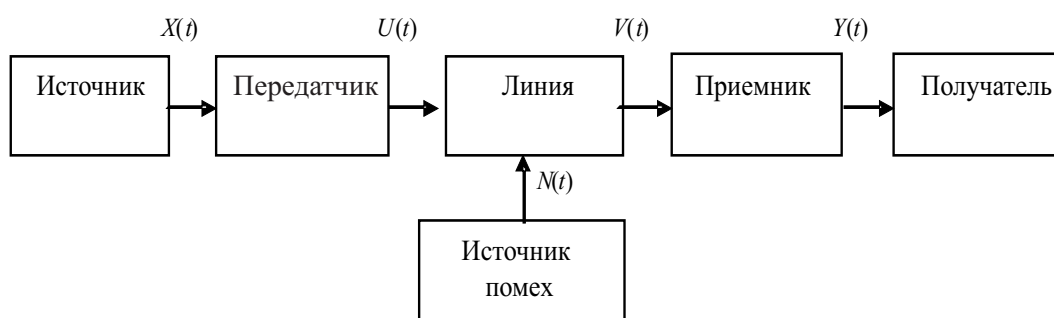
Рис. 2.1 – Укрупненная схема СПИ
