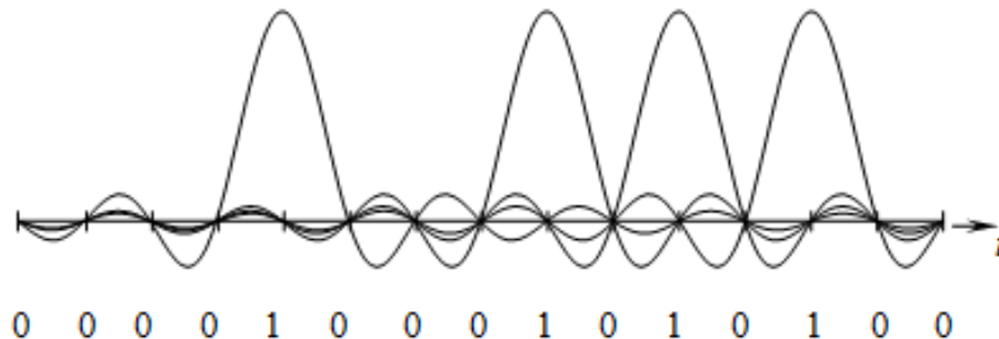
Рис. 2.15 – Слагаемые, формирующие сигнал на входе линии при передаче последовательности двоичных символов импульсами в виде функции Котельникова
