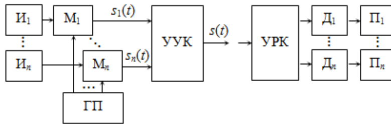
Рис. 6.1 – Упрощенная схема многоканальной СПИ
