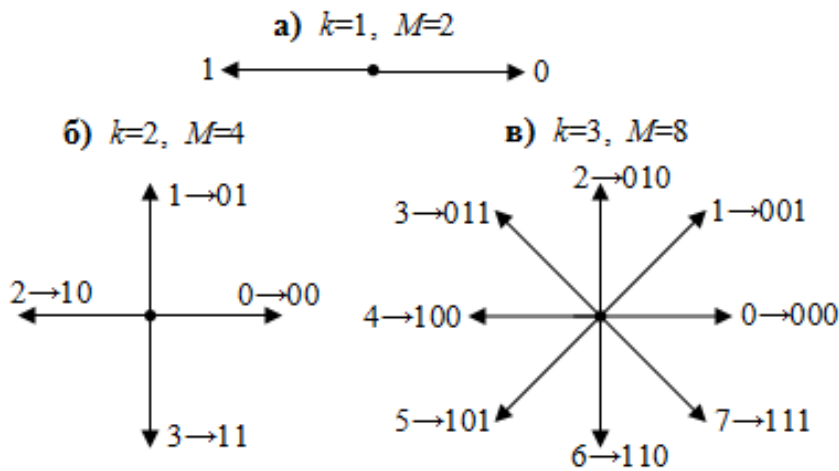
Рис. 2.18 – Векторное представление колебаний при многократной ФМ
