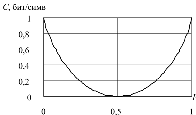
Рис. 4.5 – Пропускная способность двоичного симметричного канала без памяти
