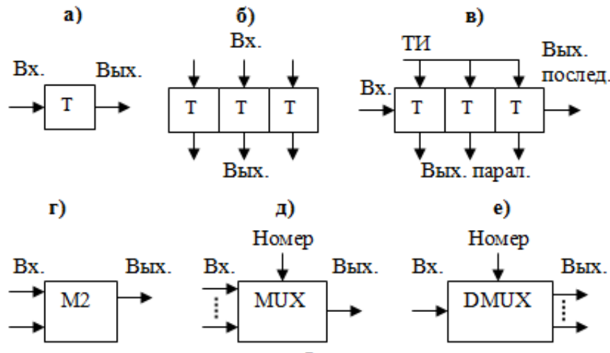
Рис. 2.2 – Элементы преобразователей сигналов:
