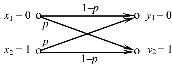
Рис. 2.21 – Переходные вероятности двоичного симметричного канала
