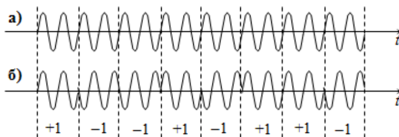
Рис. 6.8 – Преобразование информационного импульса в сигнал с внутриимпульсной ФМ: а) до преобразования; б) после преобразования.
